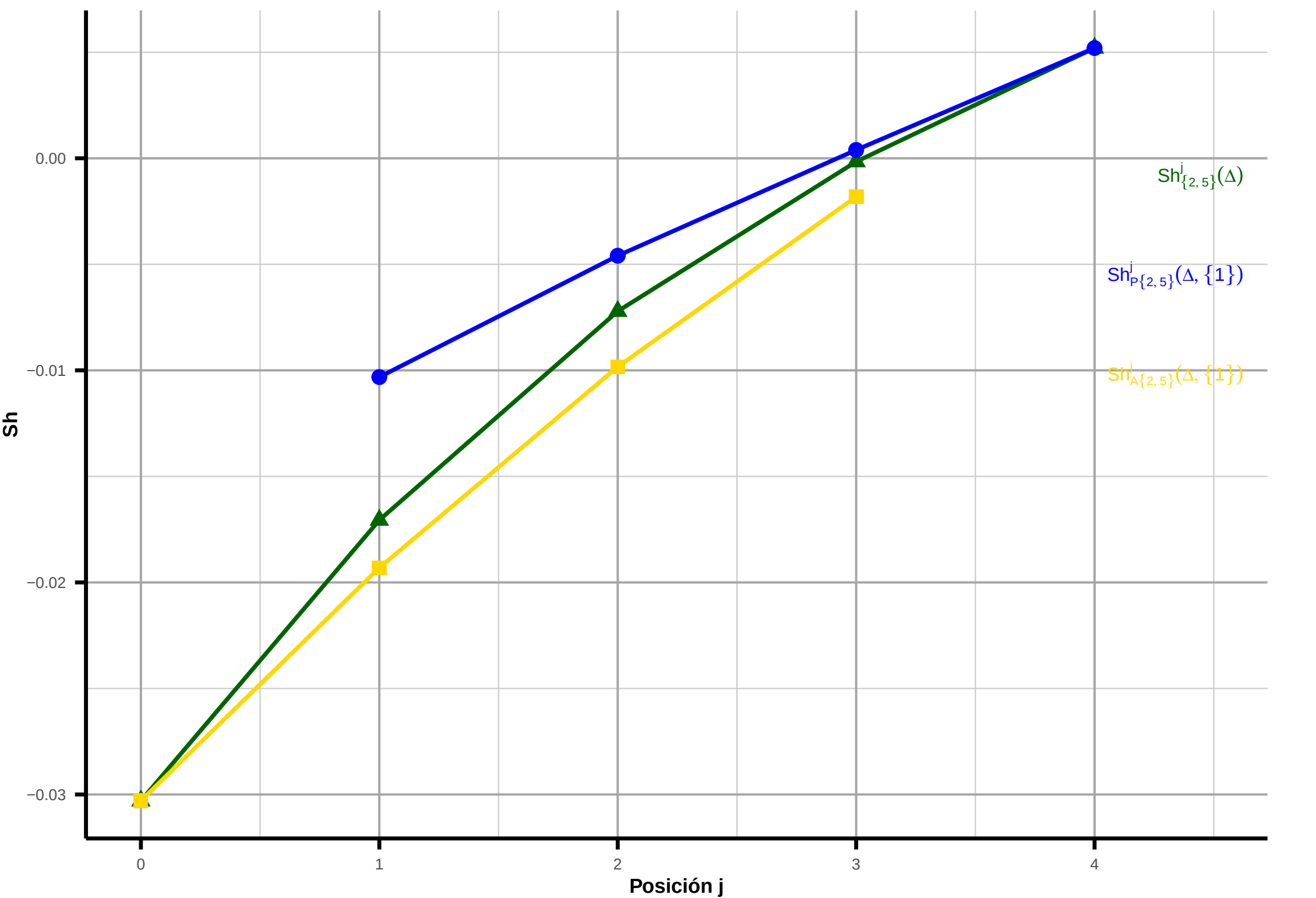
Influencia de Age [1] sobre Cho + Sex [2,5] (instancia fila = 1)
