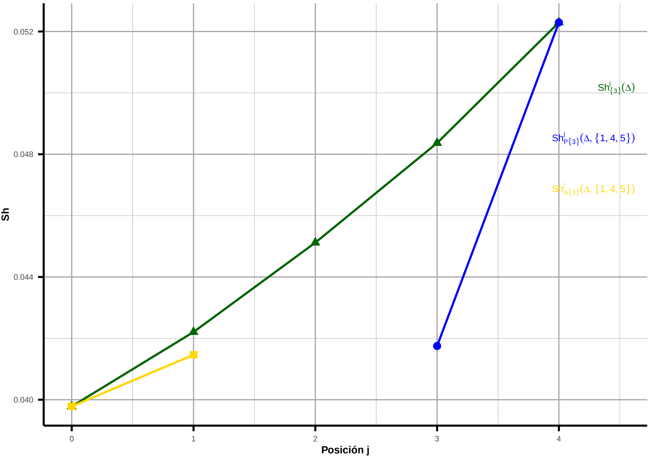
Influencia de Age + Ris + Sex [1,4,5] sobre Rac [3] (instancia fila = 1)
