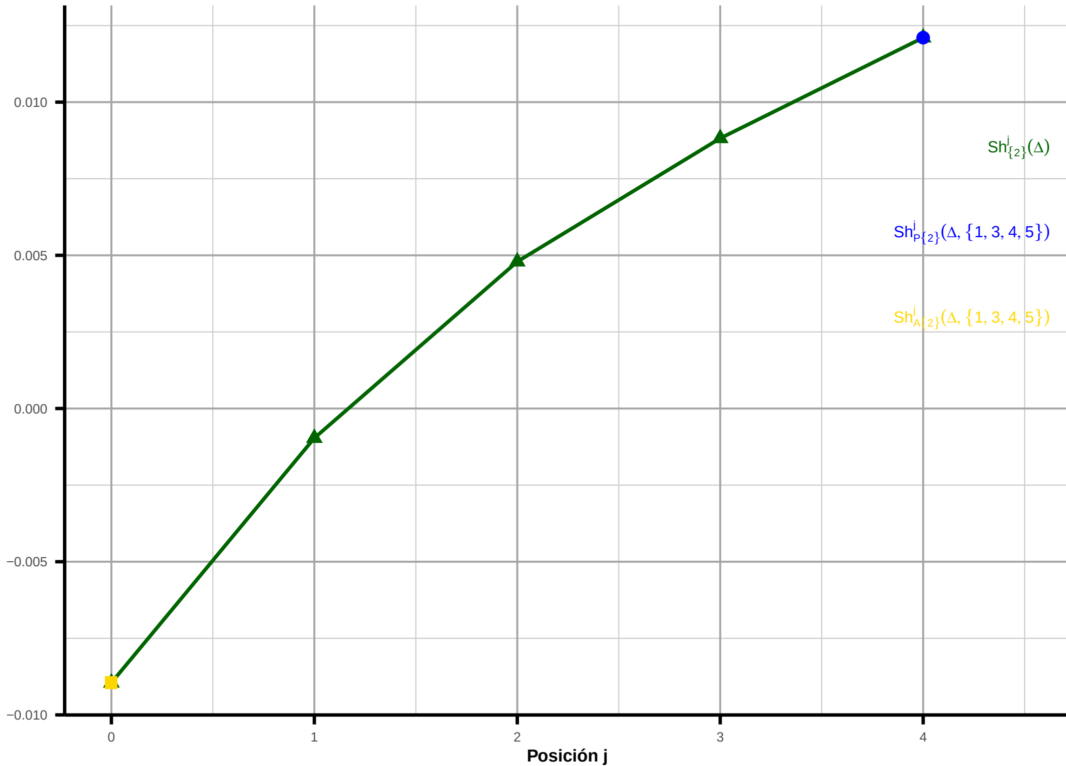
Influencia de Age + Rac + Ris + Sex [1,3,4,5] sobre Cho [2] (instancia fila = 1)
