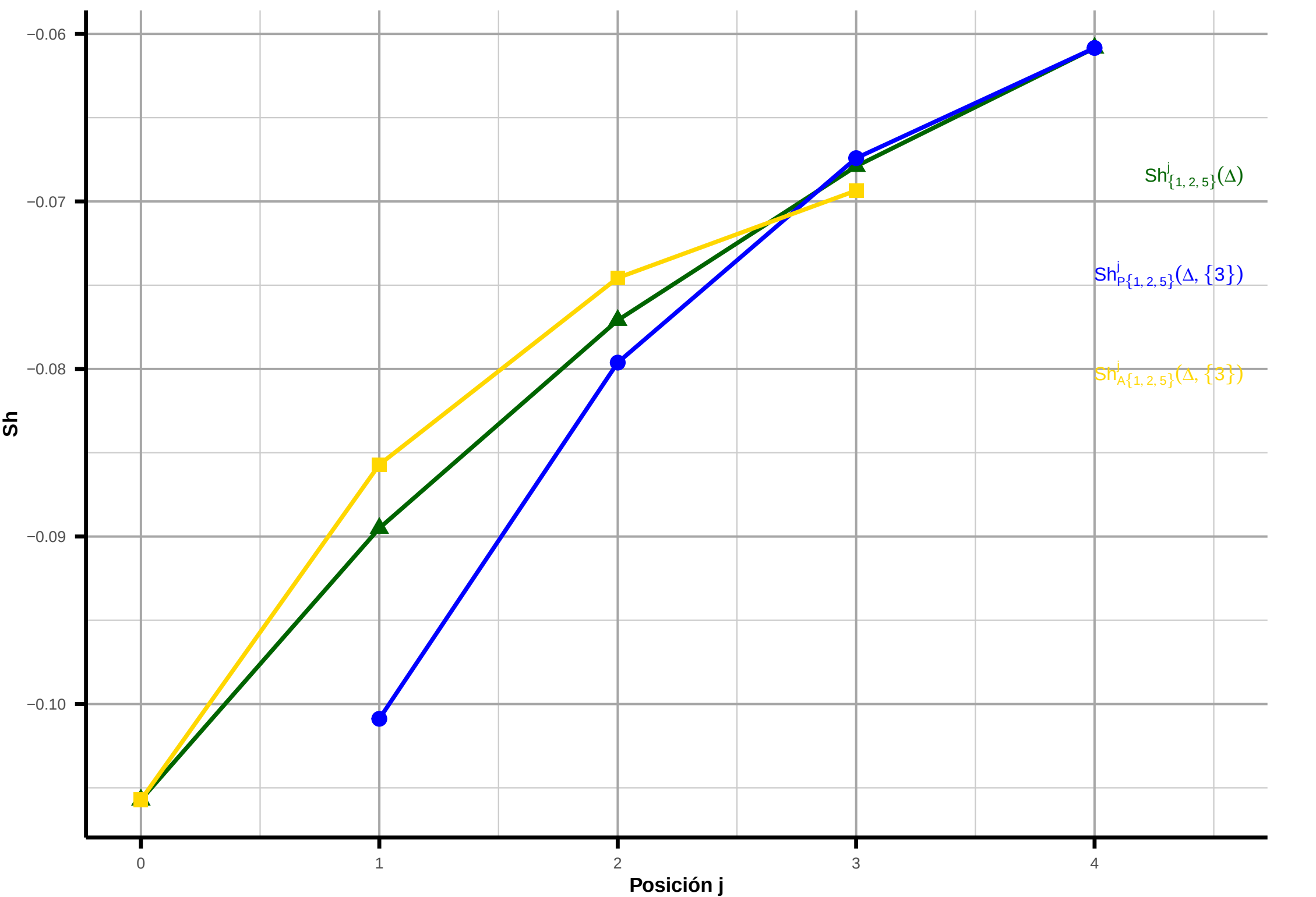
Influencia de Rac [3] sobre Age + Cho + Sex [1,2,5] (instancia fila = 1)
