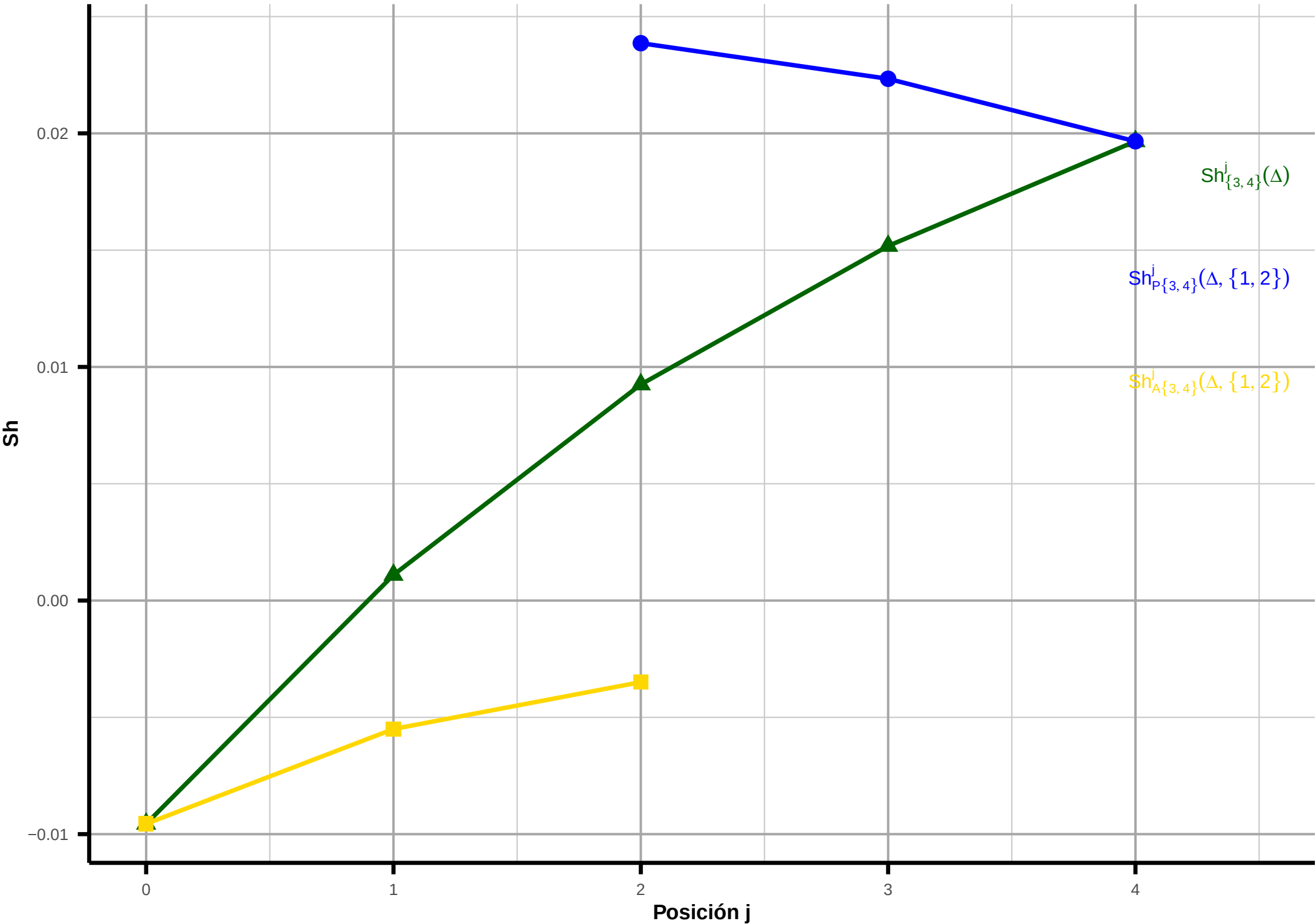
Influencia de Age + Cho [1,2] sobre Rac + Ris [3,4] (instancia fila = 1)
