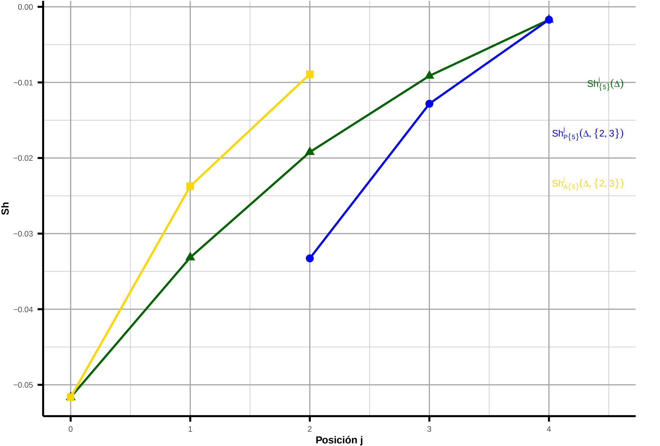
Influencia de Cho + Rac [2,3] sobre Sex [5] (instancia fila = 1)
