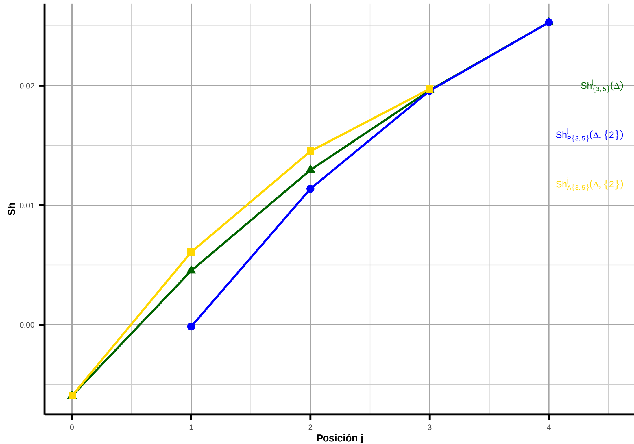
Influencia de Cho [2] sobre Rac + Sex [3,5] (instancia fila = 1)
