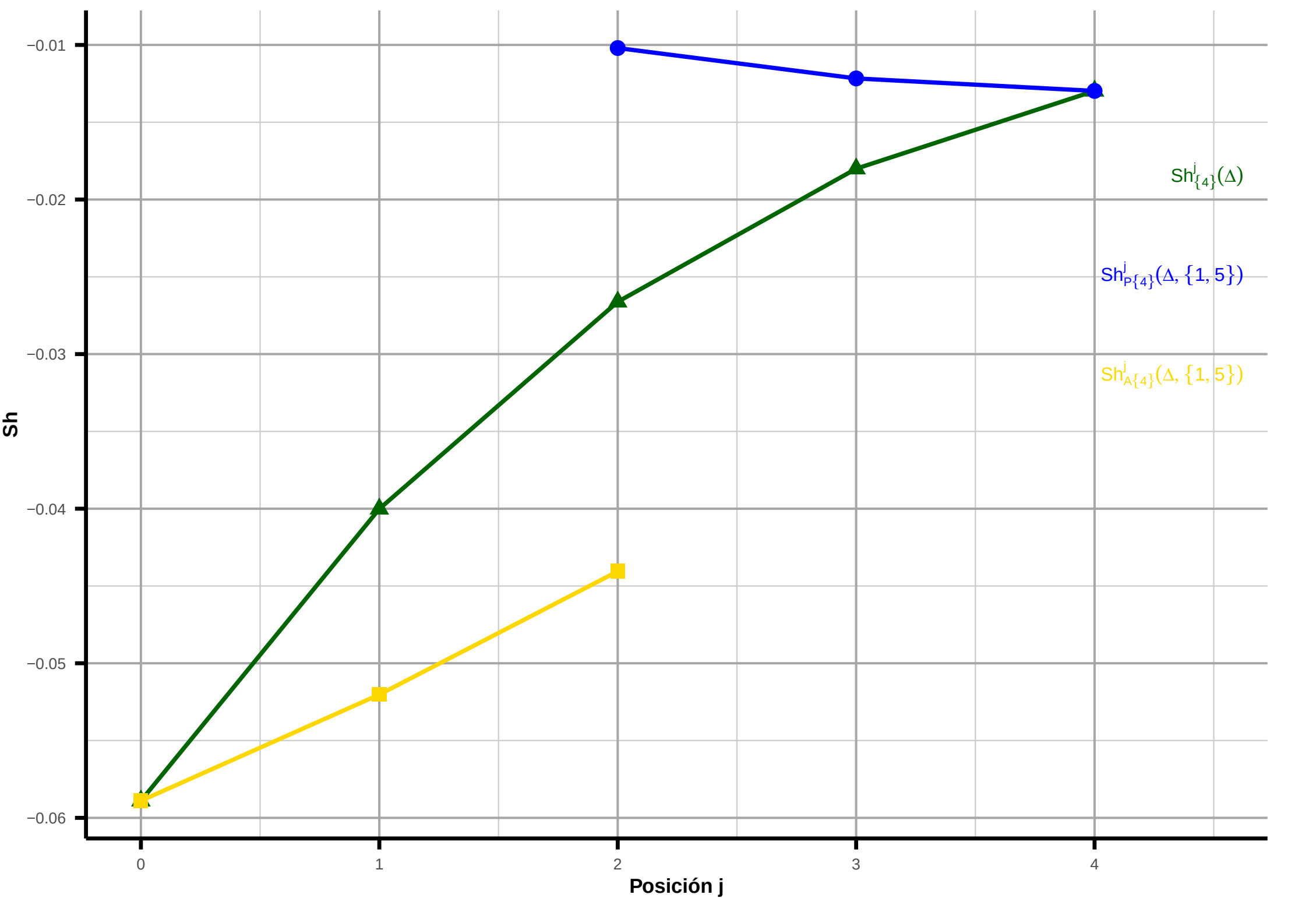
Influencia de Age + Sex [1,5] sobre Ris [4] (instancia fila = 1)
