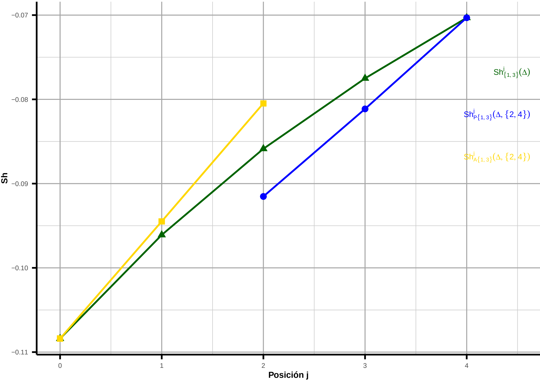
Influencia de Cho + Ris [2,4] sobre Age + Rac [1,3] (instancia fila = 1)
