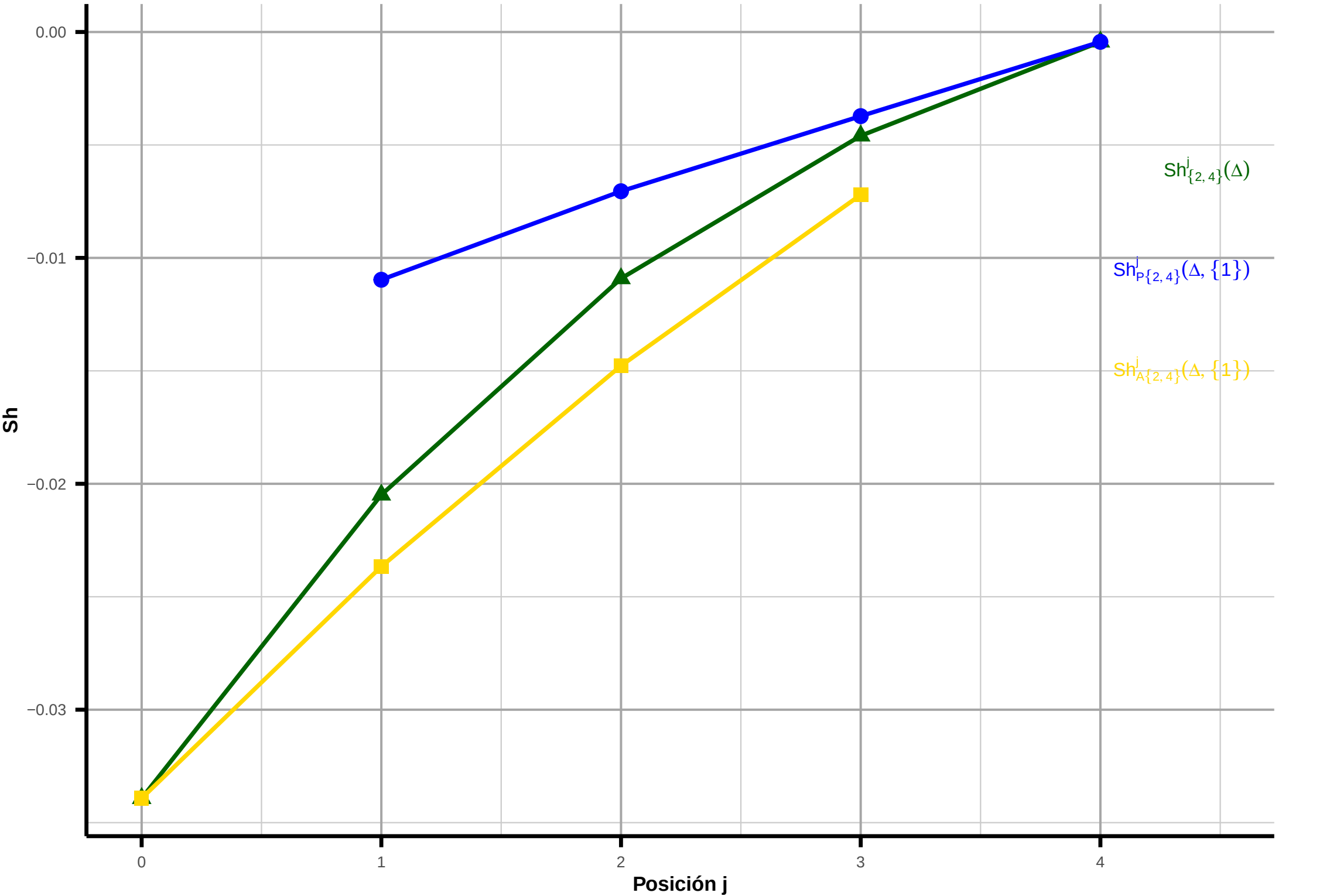
Influencia de Age [1] sobre Cho + Ris [2,4] (instancia fila = 1)
