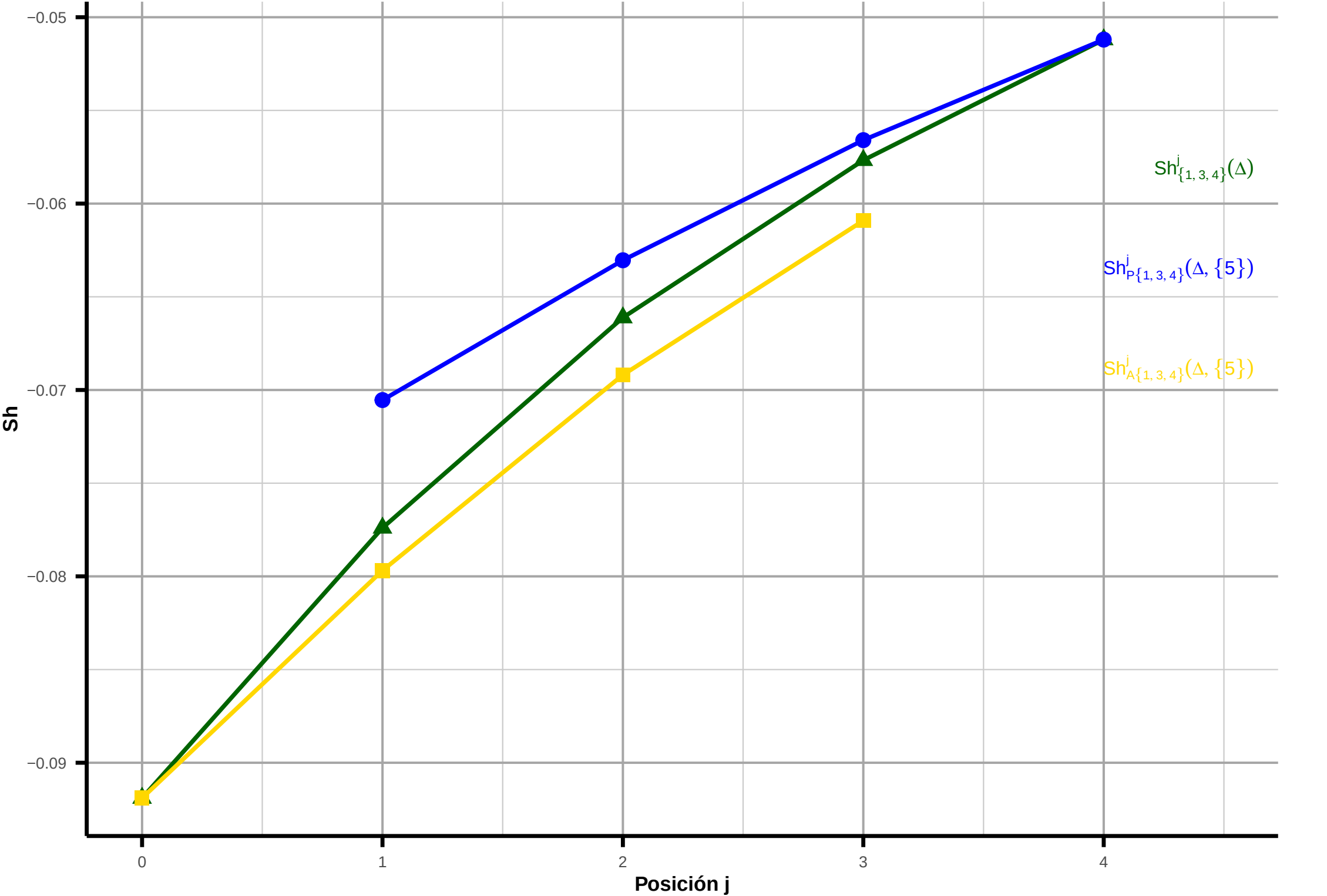
Influencia de Sex [5] sobre Age + Rac + Ris [1,3,4] (instancia fila = 1)
