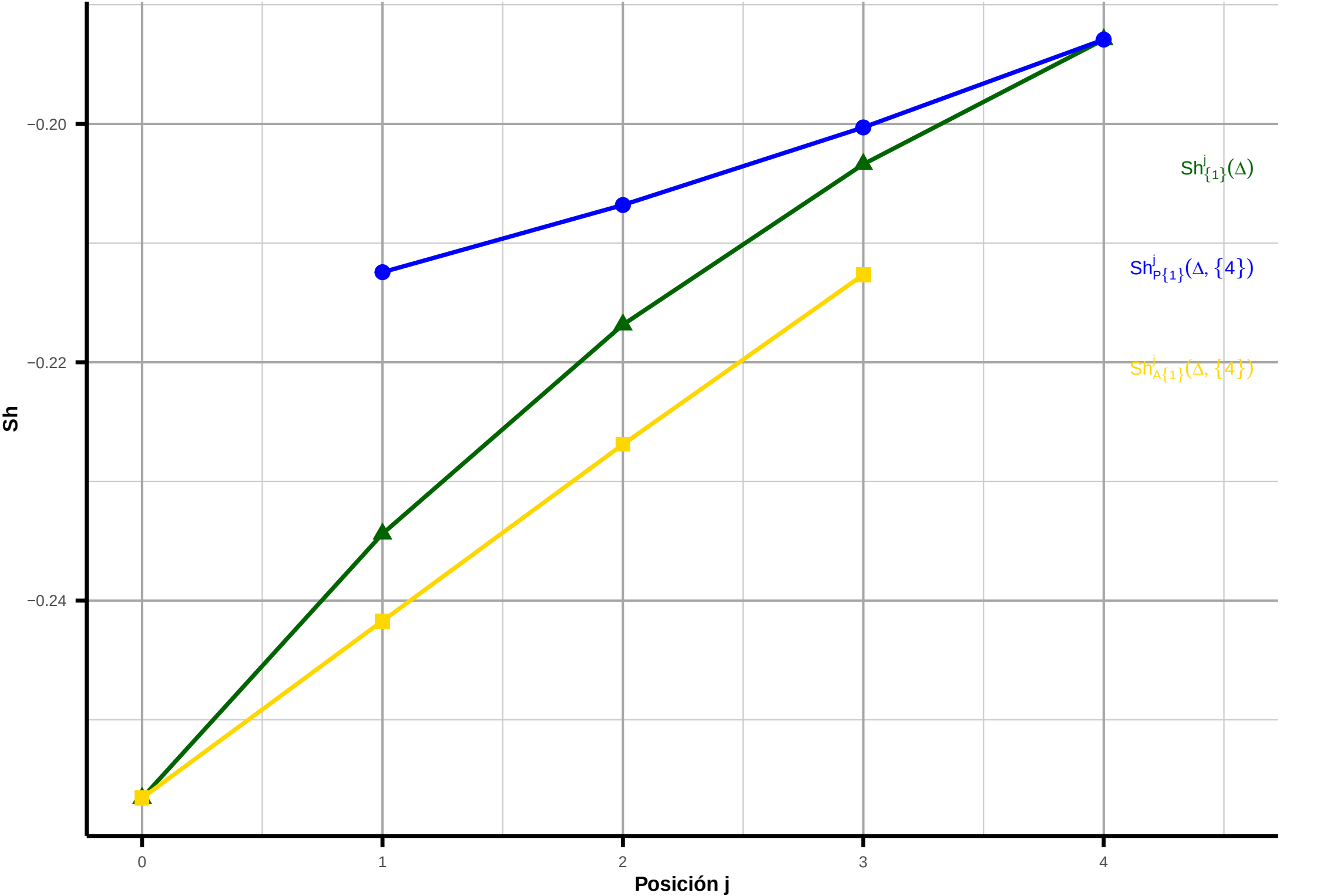
Influencia de Ris [4] sobre Age [1] (instancia fila = 1)
