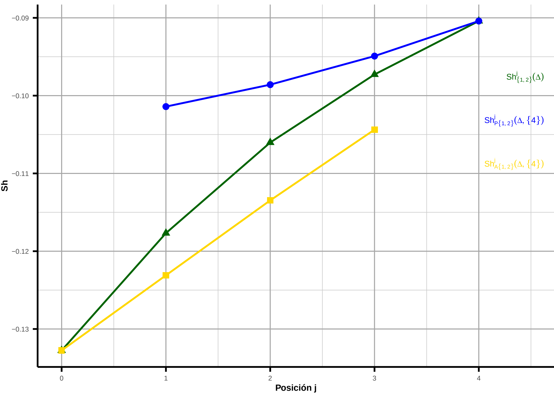
Influencia de Ris [4] sobre Age + Cho [1,2] (instancia fila = 1)
