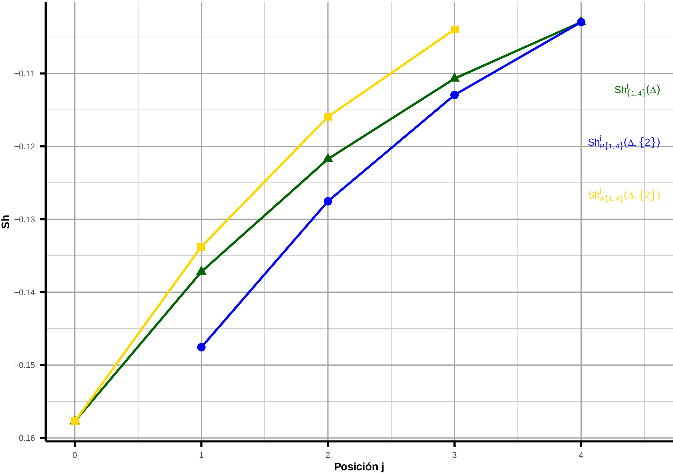
Influencia de Cho [2] sobre Age + Ris [1,4] (instancia fila = 1)
